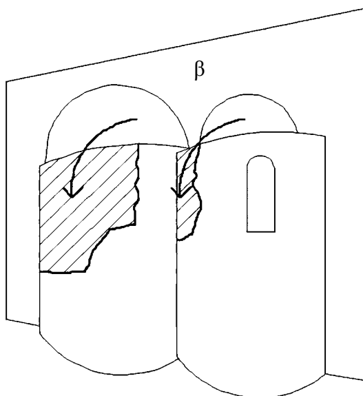
Σχήμα 9. Τοπικός μηχανισμός άνατροπής της κόγχης: (α) φωτογραφική αποτύπωση, (β) σχηματική αναπαράσταση.
