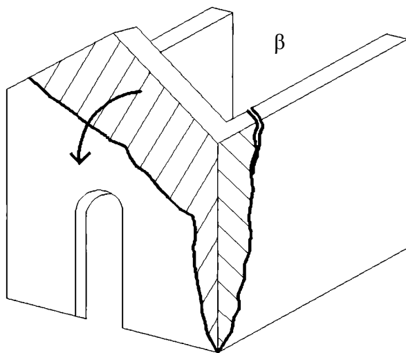
Σχήμα 8. Τοπικός μηχανισμός άνατροπής εκτός επιπέδου: α) φωτογραφική αποτύπωση, β) σχηματική αναπαράσταση.
