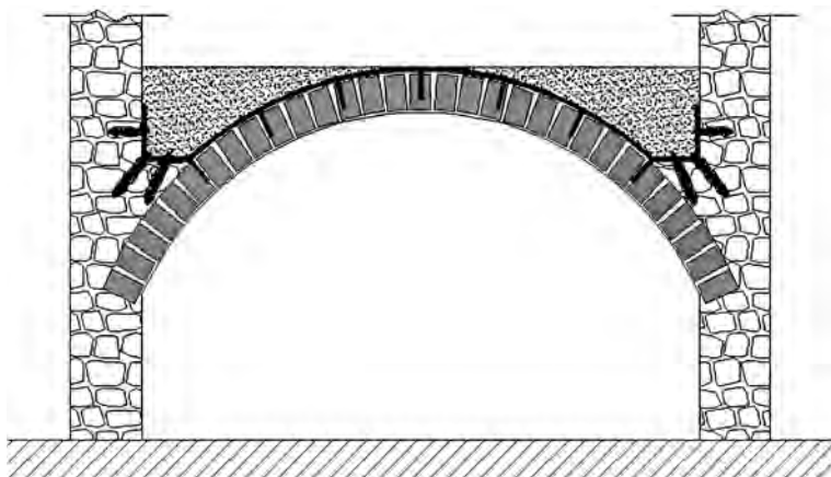
Σχήμα 6. Ενίσχυση θόλου μέ μεταλλικά στοιχεία ή μέ σύνθετα υλικά.
