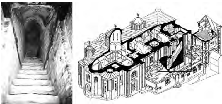
Εἰκ. 19. Ἡ ἐντὸς τῆς βόρειας τοιχοποιίας δίοδος πρὸς τὸ ὑπερῶον.
