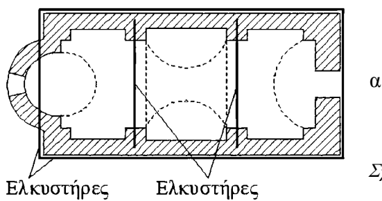
Σχῆμα 1. Συνδυασμένη μορφή άστοχίας λόγω τόσο τῆς συμπεριφοράς τῆς κατασκευῆς «ὡς συνόλου» ὅσο καὶ τῆς ἐνεργοποίησης τοπικῶν μηχανισμῶν.
