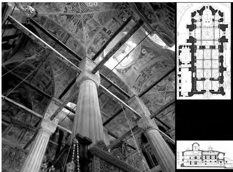
Εἰκ. 18. Ἡ Λιτή τῆς Ἱ.Μ. Δοχειαρίου Ἀγίου Ὁρους. Στὸ ἐσωτερικὸ τῆς Λιτῆς διακρίνονται δύο ἐπάλλληλες σειρές ξύλινων ἐλκυστήρων-θλιπτήρων.
