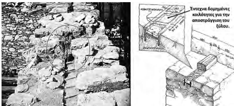
Εικ. 22. "Εντεχνα δομημένες κοιλότητες γιὰ τὴν ἀποστράγγιση τῆς ξυλοδεσιᾶς στὸν βόρειο ὀχυρωματικό τοῖχο.
