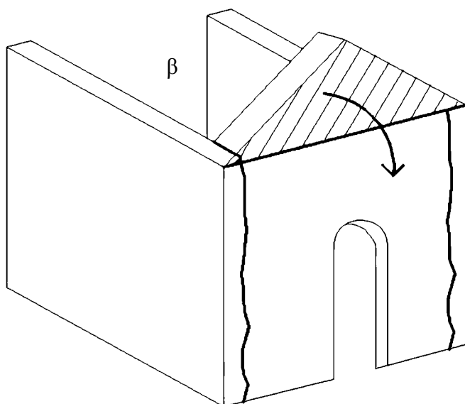
Σχῆμα 11. Ἀστοχία τοπικοῦ μηχανισμοῦ ἀνατροπῆς τυμπάνου ἀετώματος καί ἔναρξη ἀνάπτυξης τοπικοῦ μηχανισμοῦ ἀνατροπῆς δυτικῆς ὀψης: α) φωτογραφική ἀποτύπωση, β) σχηματική ἀναπαράσταση.
