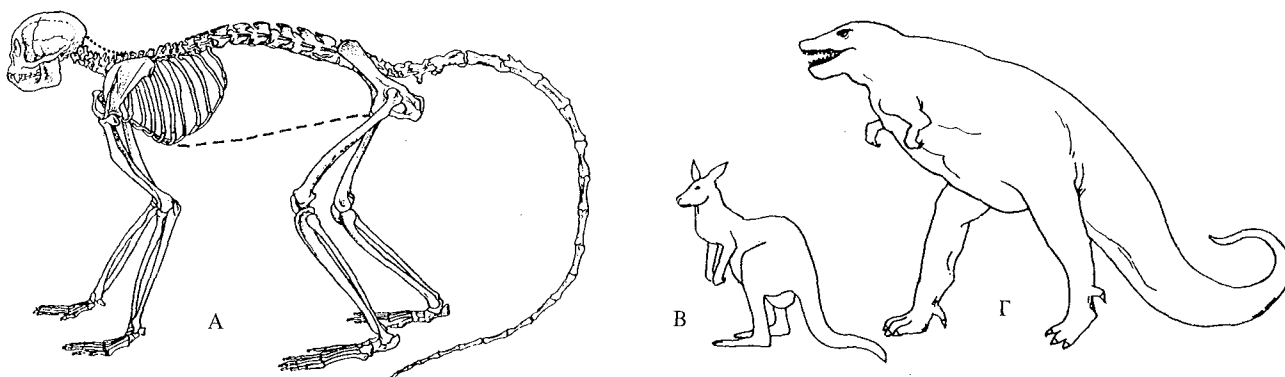
Σχῆμα 4. Στὸν τετράποδο πίθηκο (Α), τὸ κέντρο βάρους βρίσκεται στὸ πρόσθιο μέρος καὶ τὰ πρόσθια ἄκρα. Στὸ καγκουρῶ (Β) καὶ στὸν δεινόσαυρο (Γ), τὸ κέντρο βάρους βρίσκεται στὸ πίσω μέρος. Ἡ διποδία τους ἐνισχύεται μὲ μιὰ βαριὰ καὶ δυνατὴ οὐρά.
