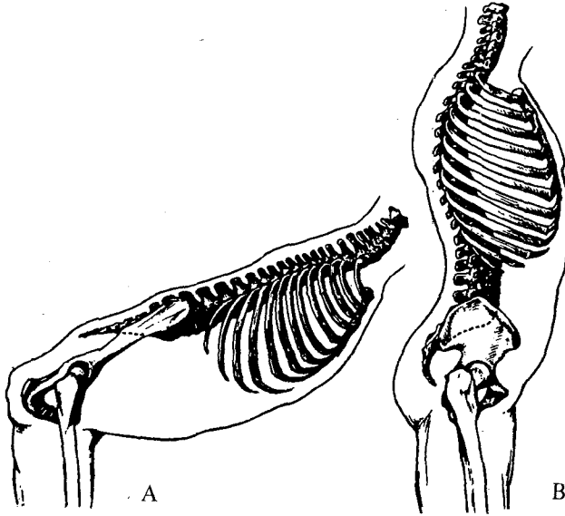
Σχήμα 5. Λεκάνη χιμπαντζή (A) και ανθρώπου (B). Άξιοσημείωτη ή διαφορά του σχήματος και του μεγέθους της λεκάνης, καθώς και η σχέση ανάμεσα στη λεκάνη, τη σπονδυλική στήλη και το μηριαίο όστον.
