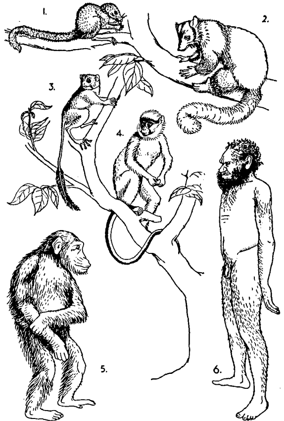
Σχήμα 6. Σειρά ζώντων ειδών αρχαιότερων πρωτευόντων, που υποτίθεται ότι συνδέουν ανατομικώς τον άνθρωπο με μερικά από τα πιό πρωτόγονα πλακουντοφόρα θηλαστικά: 1. σκίουρος 2. λεμούρ 3. μικρός λεμούρ 4. πίθηκος 5. χιμπαντζής 6. Αυστραλός ιθαγενής.
