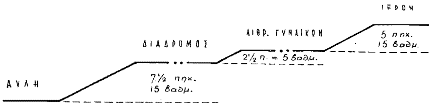
Σχ. 17. Κατὰ μήκος τομὴ βαθμίδων τῶν διαδοχικῶν αἰθρίων τοῦ Ναοῦ [τοῦ Ἡρώδου κατὰ Wolff. (Πρωτότυπον σχέδιον).
