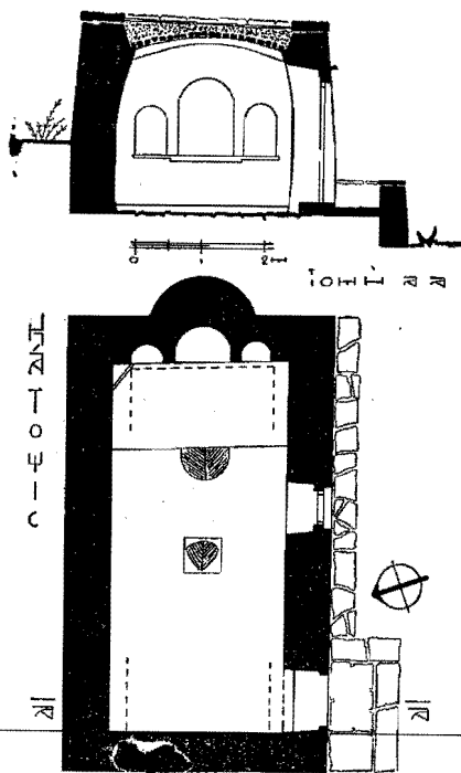
Εἰκ. 7. Ἡ κάτοψις καὶ ἡ κατὰ πλάτος τομὴ τῆς μικρᾶς βασιλικῆς τῶν ἁγίων Πάντων παρὰ τὸ χωρίον Κάστρο τῆς νήσου Σίφνου.
