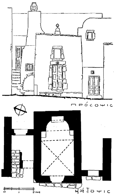
Εἰκ. 13. Ἡ κάτοψις καὶ ἡ πρόσοψις τοῦ ναῖσκου τοῦ Θεολόγου (τὸ «Θεολοκία») εἰς Νιμπορζιὰ Σαντορίνης.
