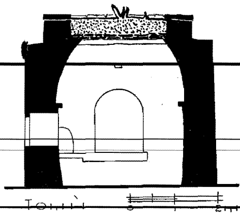
Εἰκ. 6. Ἡ κατὰ πλάτος τομὴ τοῦ ναοῦ τῶν Εἰσοδίων τῆς Θεοτόκου ἐν Ἀντιπάρφ.
