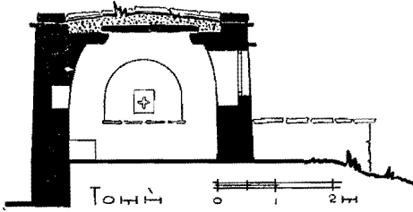
Εἰκ. 8. Ἡ κατὰ πλάτος τομὴ τοῦ ναοῦ τῆς ἁγίας Τριάδος εἰς Μαΐνητες Ἄνδρου.
