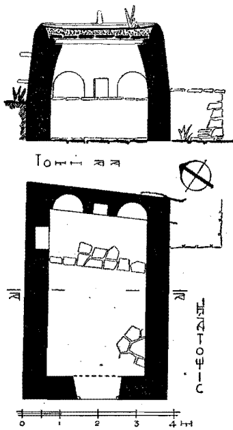
Εἰκ. 4. Ἡ κάτοψις, καὶ ἡ κατὰ πλάτος τομὴ τοῦ ἐρημοκκλησίου τοῦ ἁγίου Νικολάου εἰς θέσιν «Βορεινῆς» Κύθου.
