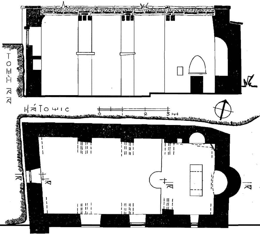
Εἰκ. 20. Ἡ κάτωψις καὶ ἡ κατὰ μῆκος τομὴ τῶν ἁγίων Ἀναργύρων εἰς τὸ χωρίον Ἀρνάδος τῆς Ἱήνου.
