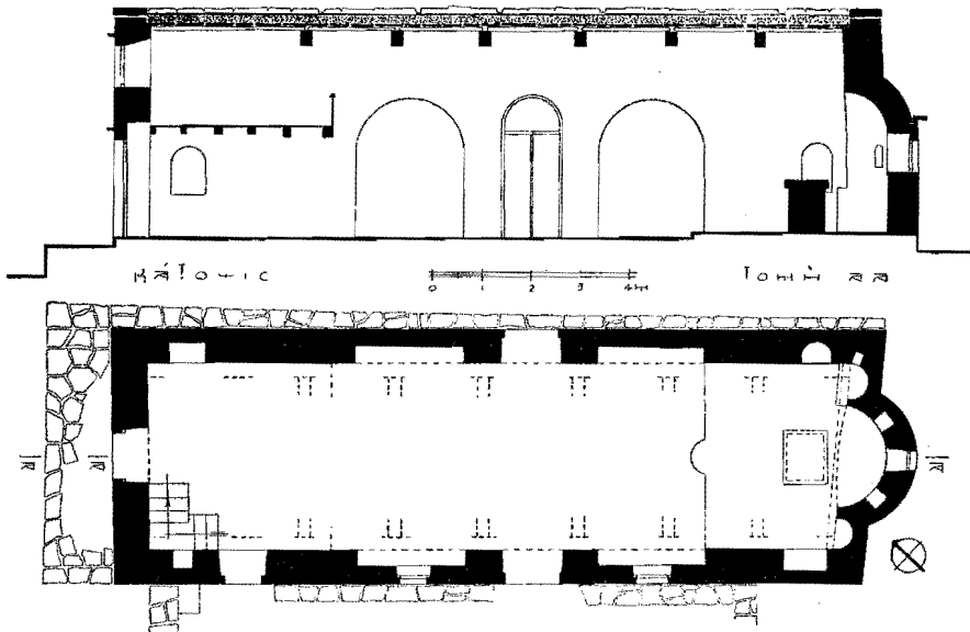
Εἰκ. 14. Ἡ κάτοψις καὶ ἡ κατὰ μῆκος τομὴ τοῦ ναοῦ τοῦ ἁγίου Λουκά εἰς τὸν Ἀρτεμιῶνα Σίφνου.
