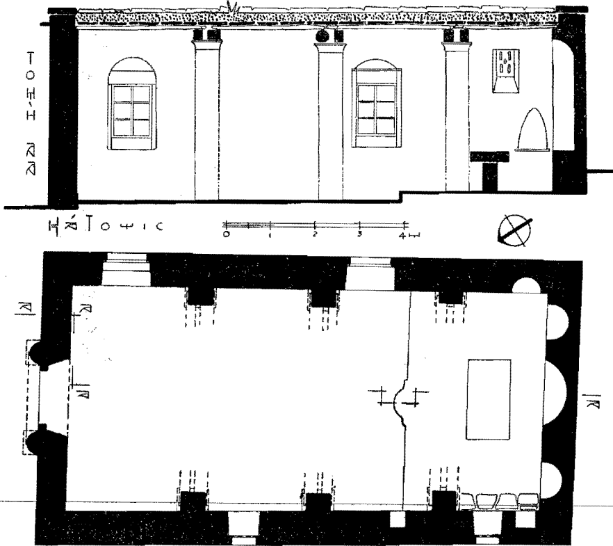
Εἰκ. 15. Ἡ κάτωφωσις καὶ ἡ κατὰ μῆκος τομὴ τοῦ ναοῦ τοῦ ἀγίου Γεωργίου εἰς τὸν Πύργον τῆς νήσου Τήνου.
