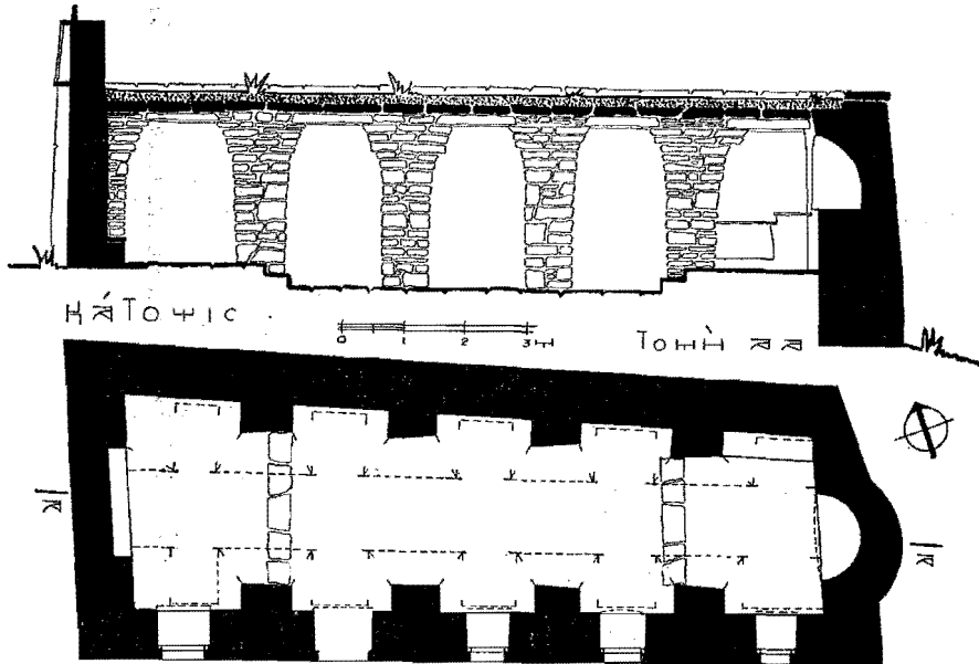
Εἰκ. 18. Ἡ κάτοψις καὶ ἡ κατὰ μῆκος τομὴ τοῦ Ταξιάρχου εἰς τὸν Τριαντάρο Τήνου.
